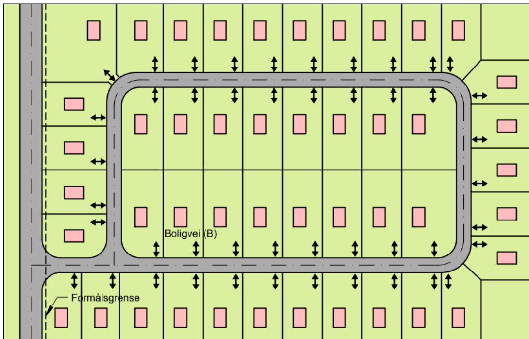
Figur 4.17: Lang boligvei (B) i sløyfe
