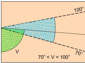
Figur 4.25: Anbefalte vinkler for T-kryss
