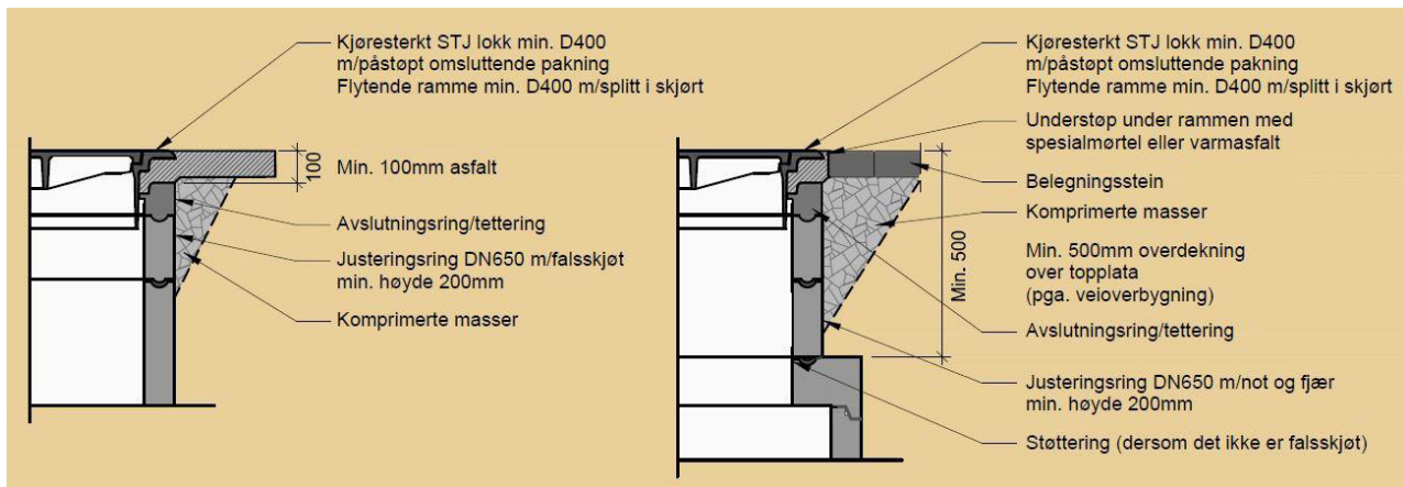
Figur 6.9: Detalj for asfaltering ved kumlokk i flyteramme
