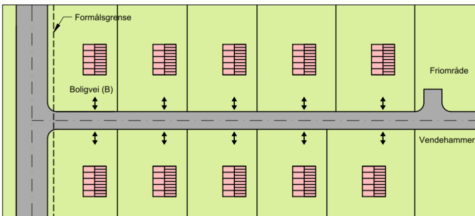
Figur 4.16: Kort boligvei (B) med snuplass
