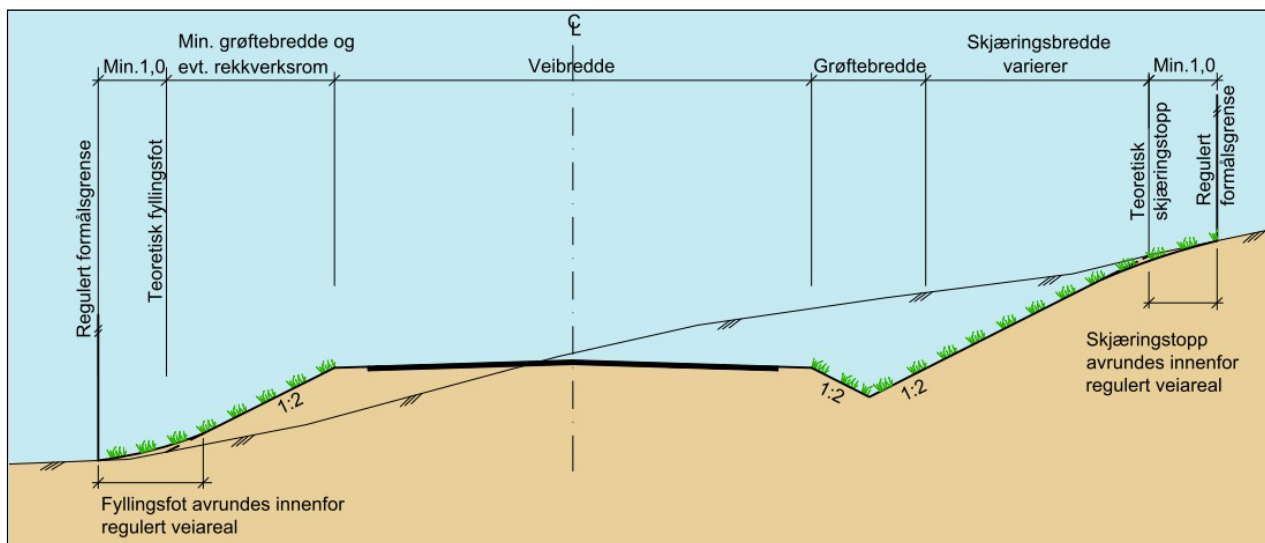
Figur 4.5: Prinsipp for reguleringsgrense der vei ligger i skjæring og fylling
