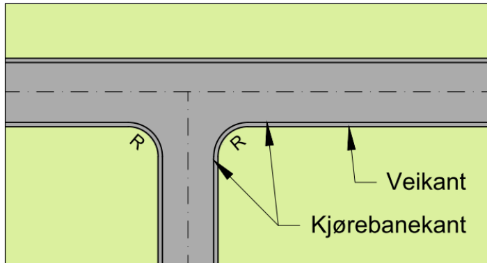
Figur 4.28: Tilslutningsradier mellom kjørebane kantene i et veikryss
