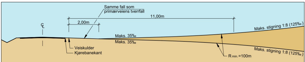
Figur 4.32: Tillatt lengdeprofil for atkomstvei i veikryss
