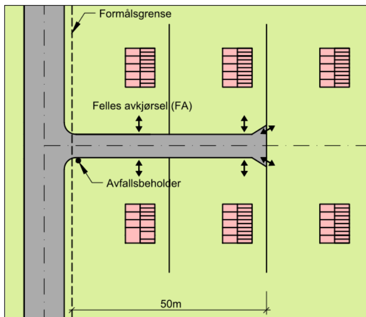
Figur 4.12: Felles avkjørsel (FA1)
