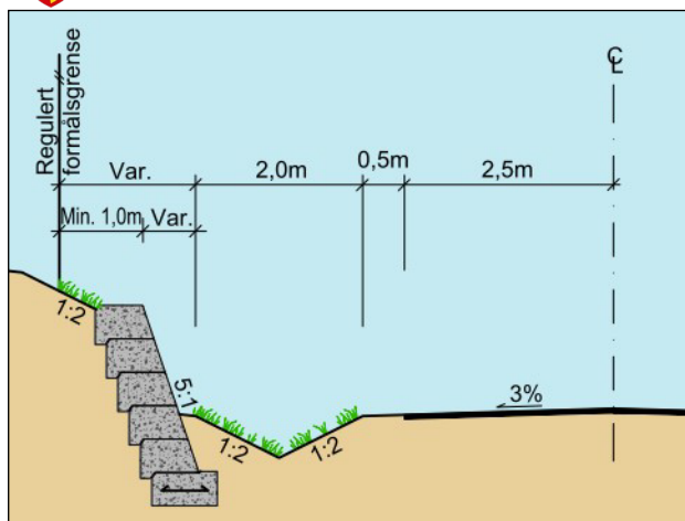
Figur 4.2: Prinsipp for reguleringsgrænse der mur skal være en del av veiens eiendom
