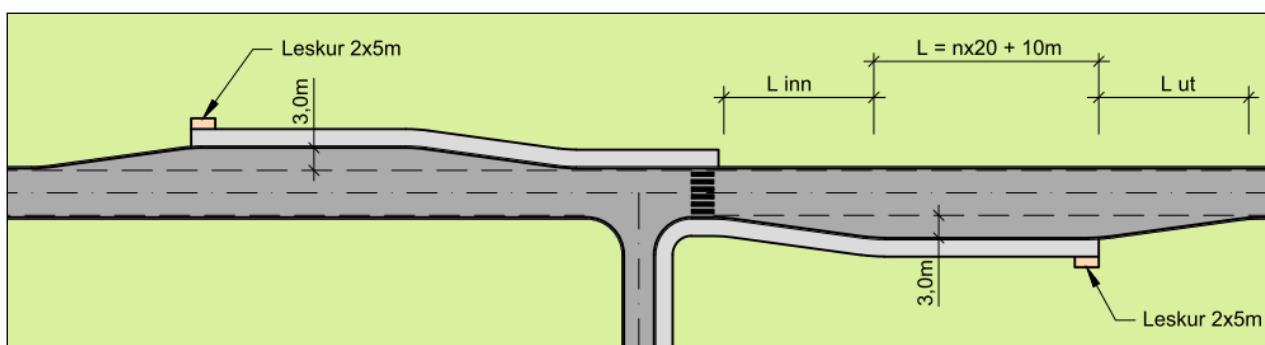
Figur 4.41: Utforming av busslomme (n= antall busser)
