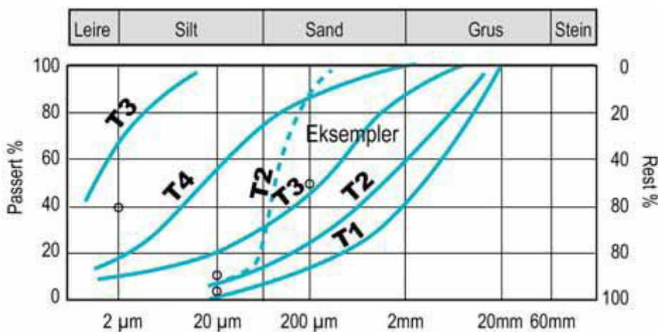
Figur 6.4: Kornfordelingskurver
