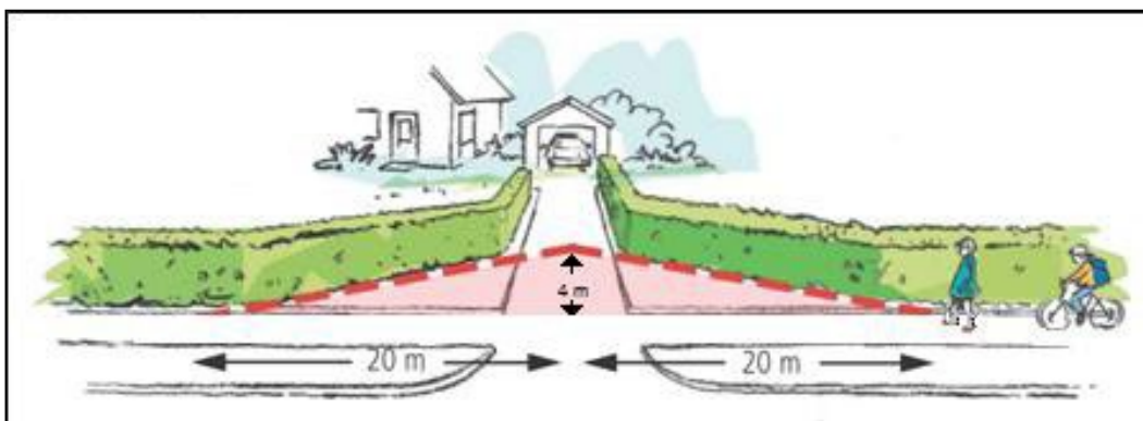
Figur 4.35: Eksempel på frisiktzone boligavkjørsler
