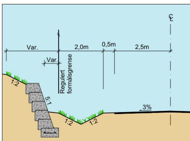
Figur 4.3: Prinsipp for reguleringsgrænse der mur skal være en del av privat eiendom
