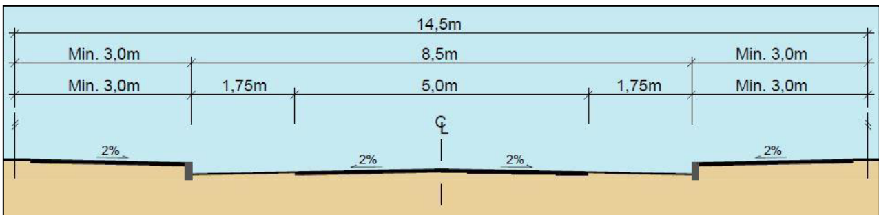
Figur 4.20: Tverrprofil for atkomstgate (AG) med to-sidig sykkelfelt
