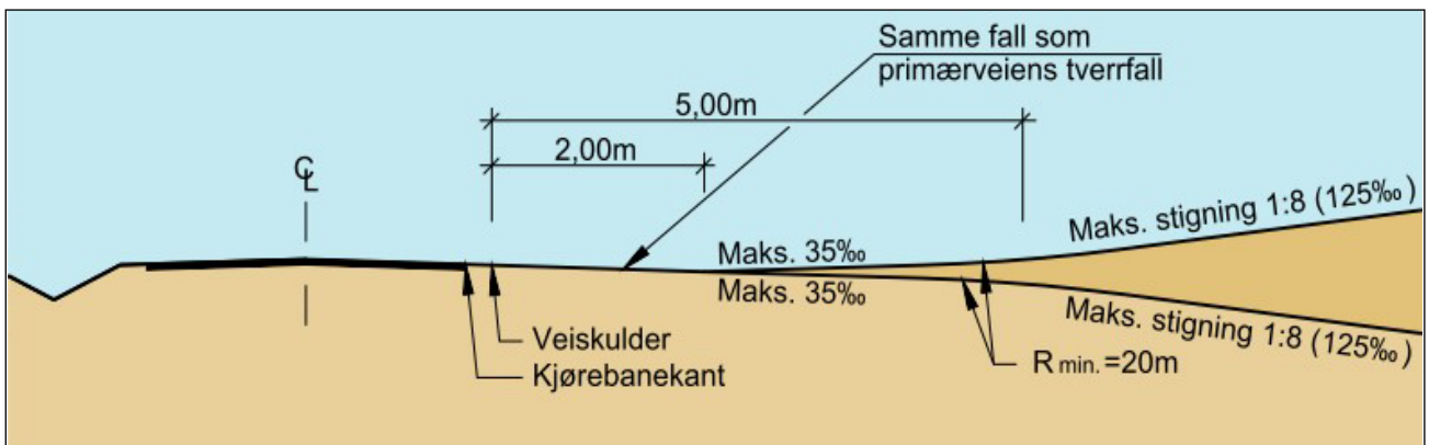
Figur 4.30: Tillatt lengdeprofil for felles avkjørsel mot annen vei
