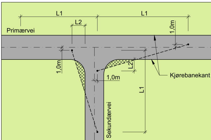
Figur 4.37: Frisiktsoner
