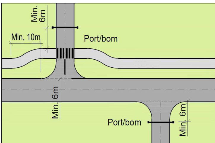
Figur 4.27: Plassering av porter og bommer langs vei og gang- og sykkelvei
