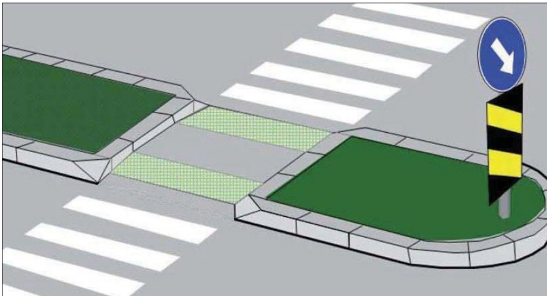
Figur 5.3 Trafikkøyer eller midtdeler utføres med lysåpningsbredde på 3,0m med dekke i plan
