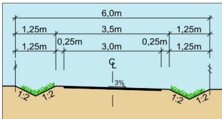
Figur 4.13: Tverrprofil for felles avkjørsel (FA1)
