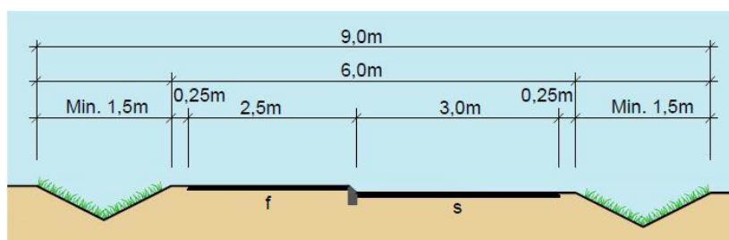
Figur 4.11: Typisk snitt av sykkelveg med fortau
