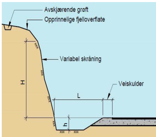
Figur 6.1: Utforming av fanggrøft mellom skjæring og vei
