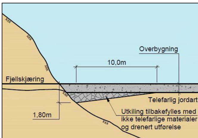
Figur 6.2: Prinsipp for overgang mellom fjellskjæring og telefarlig grunn
