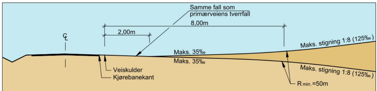
Figur 4.31: Tillatt lengdeprofil for boligvei i veikryss
