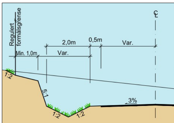
Figur 4.1: Prinsipp for reguleringsgrense ved fjellskjæring
