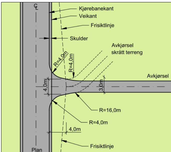
Figur 4.29: Utforming av avkjørsler og kryss
