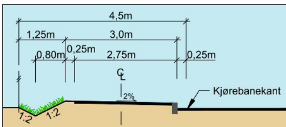
Figur 4.8: Tverrprofil fortau (F)
