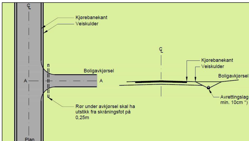
Figur 6.8: Stikkrenne
