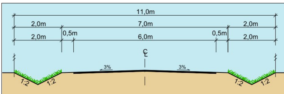
Figur 4.19: Tverrprofil for samlevei (S)
