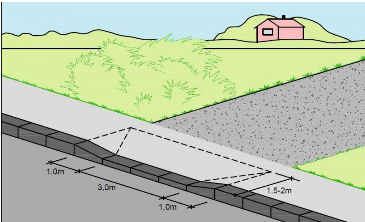
Figur 4.34: Privat boligavkjørsel krysser fortau.
