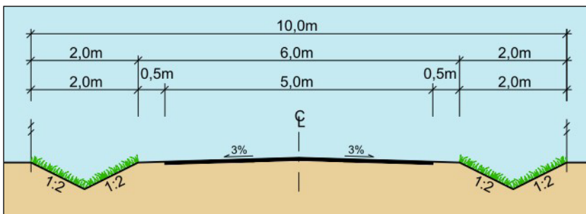
Figur 4.18: Tverrprofil for adkomstvei (A)
