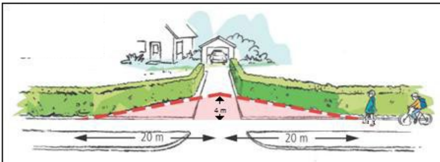
Figur 4.36: Eksempel på frisiktzone
