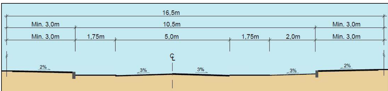
Figur 4.21: Tverrprofil for atkomstgate med kantparkering, her vist med to-sidig sykkelfelt og ensidig kantparkering
