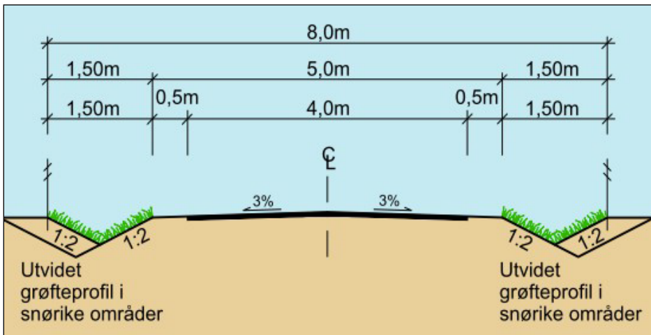
Figur 4.15: Tverrprofil for boligvei (B)
