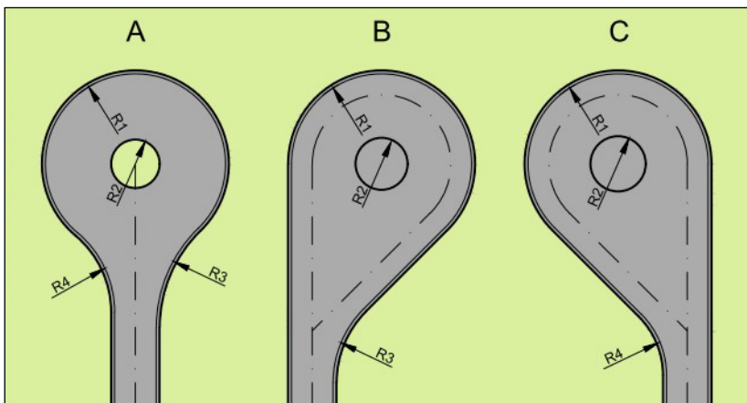
Figur 4.39: Utforming av snuplasser
