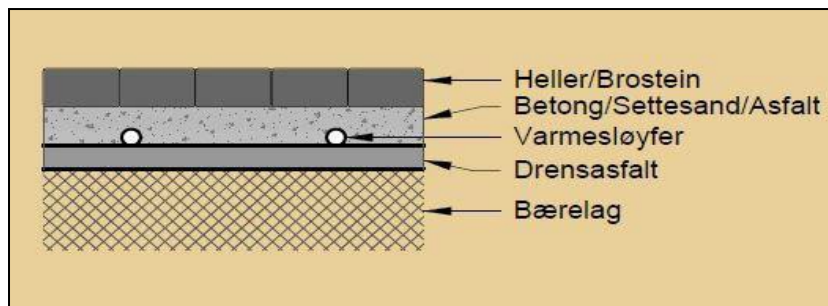
Figur 6.7: Prinsipp for overbygning med gatevarme.
