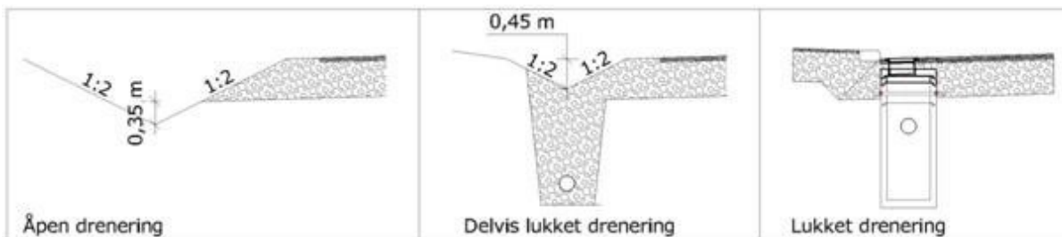
Figur 5.1: Prinsipp for utforming av drencsystem
