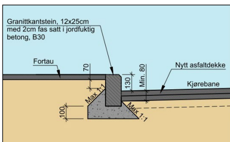
Figur 5.2: Detalj av kantstein
