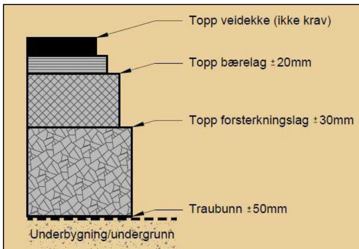
Figur 6.6: Toleransekrav i overbygningen
