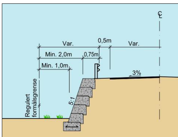
Figur 4.4: Prinsipp for reguleringsgrænse der mur bygger opp veien som en del av veianlegget
