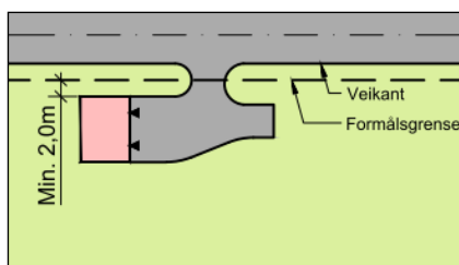
Figur 4.6: Garasje parallelt med vei
