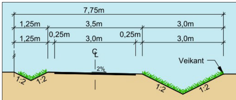
Figur 4.9: Tverrprofil gang- og sykkelvei langs kjørevei
