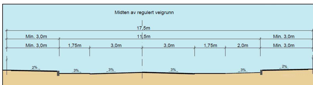
Figur 4.22: Tverrprofil for samlegate, her vist med tosidig sykkelfelt og ensidig kantparkering
