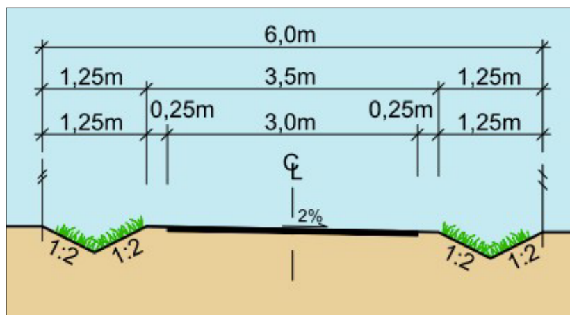
Figur 4.9: Tverrprofil gang- og sykkelvei langs kjørevei
