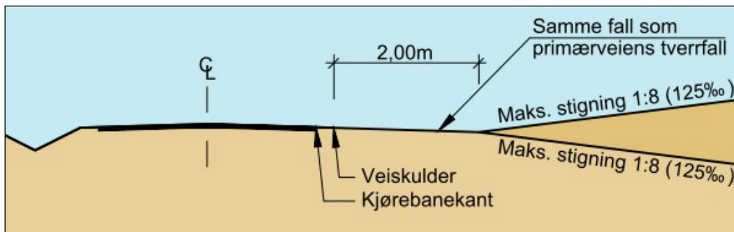
Figur 4.33: Tillatt lengdeprofil for boligavkjørsel mot annen vei
