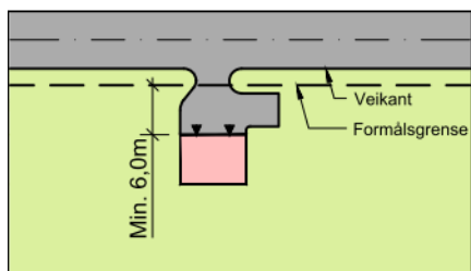
Figur 4.7: Garasje, vinkelrett på vei
