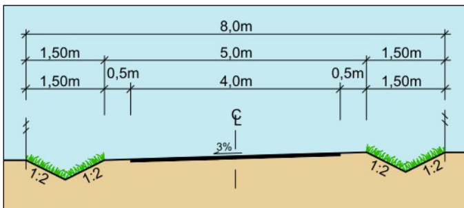
Figur 4.14: Tverrprofil for felles avkjørsel for 13 - 80 boenheter (FA2)
