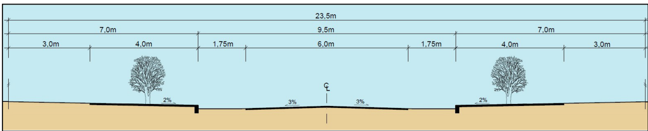
Figur 4.23: Tverrprofil for hovedgate med tosidig sykkelfelt
