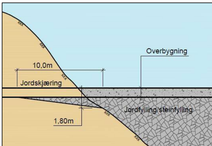
Figur 6.3: Prinsipp for overgang mellom jordskjæring og fylling
