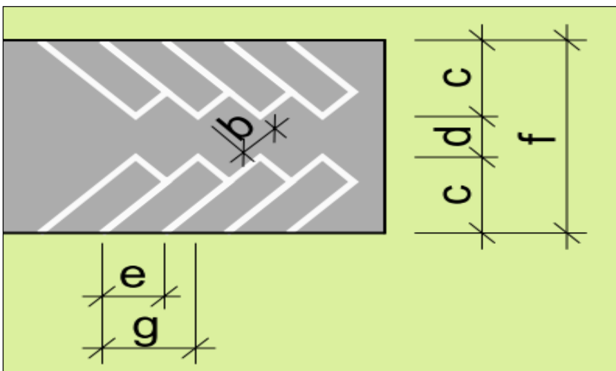
Figur 4.43: Utforming av generell parkeringsplass
