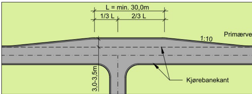
Figur 4.38: Utforming av passeringsfelt
