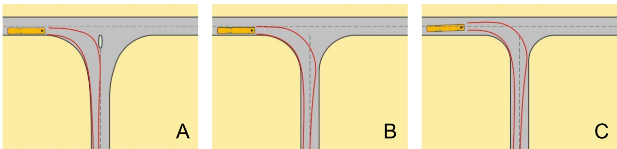
Figur 4.24: Dimensjonerende kjøremåte A, B og C
