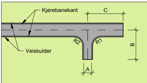
Figur 4.40: Utforming av vendehammer
