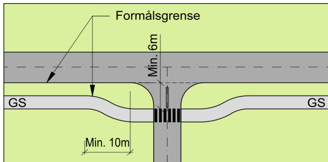
Figur 4.26: Anbefalt utforming av kryssing mellom gang- og sykkelvei og T-kryss
