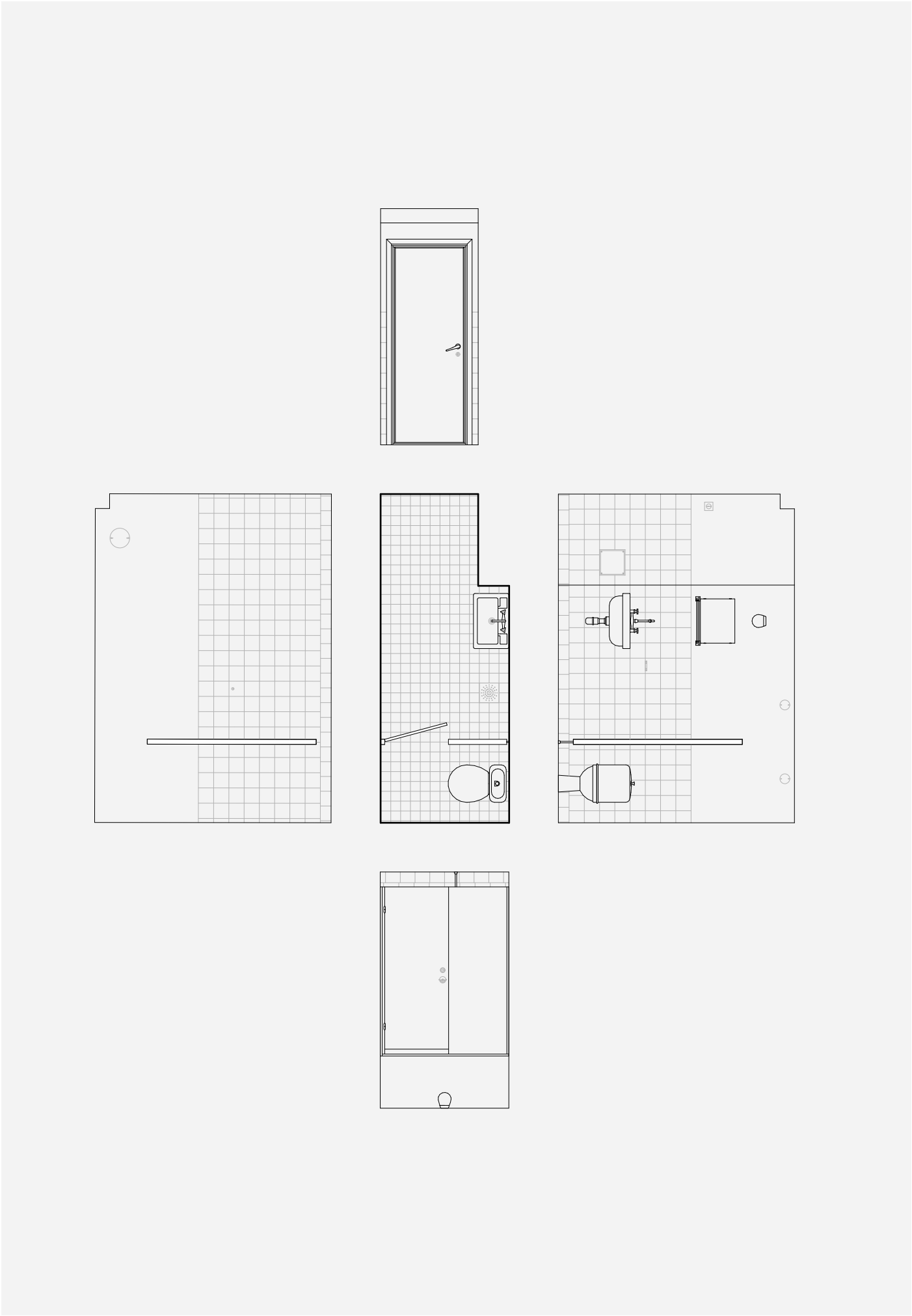
Skjemateikning av toalett i 3. etasje i kontorfløya 1:50
